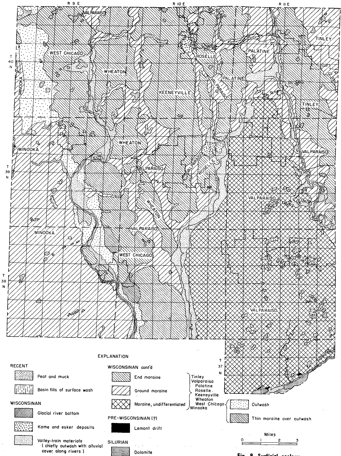
Fig. 8. Surficial geology.
